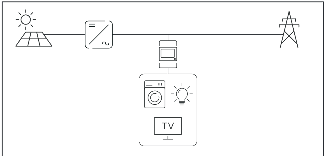
SO-mittari kulutushaarassa
